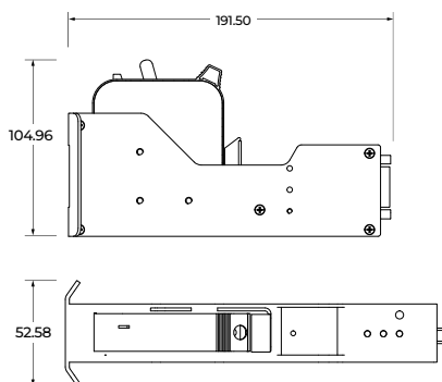
MAXe Printhead
